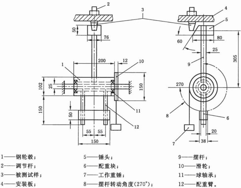
图 1 碰撞试验设备示意图
